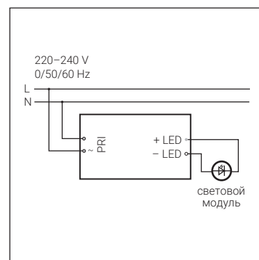
Схема подключения
